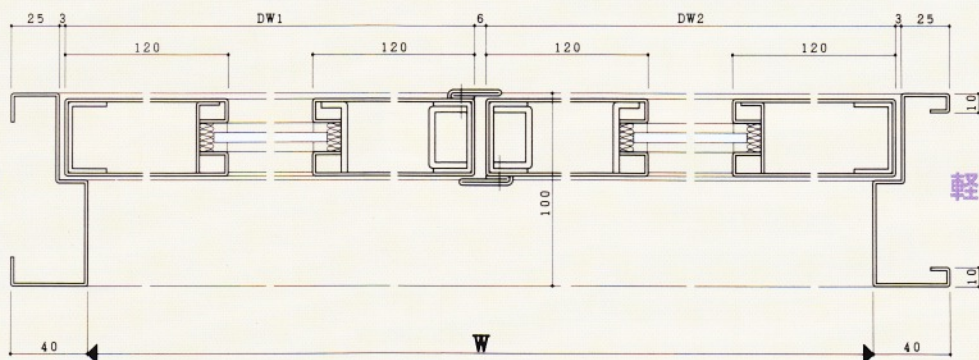
両開き
