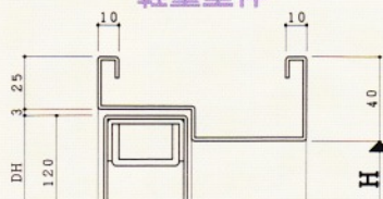
軽量壁枠
