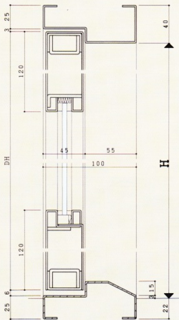
RC枠
