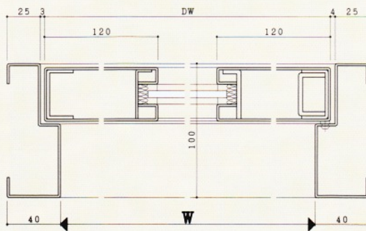
両開き
